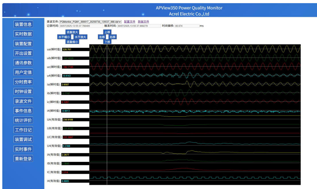
图 1.5 波形界面
