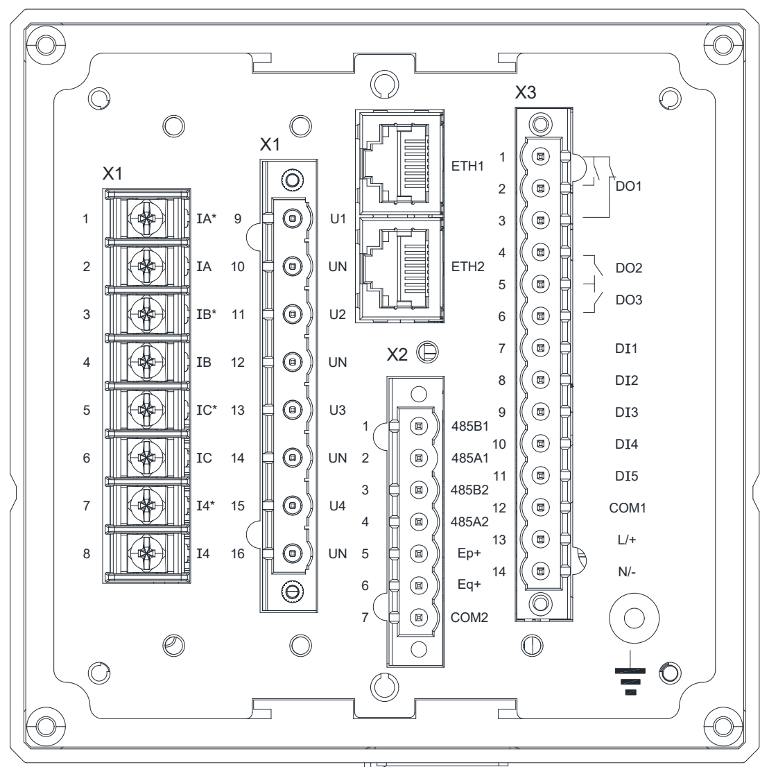
图 3.3 背部端子图 Fig. 3.3 Back terminals
