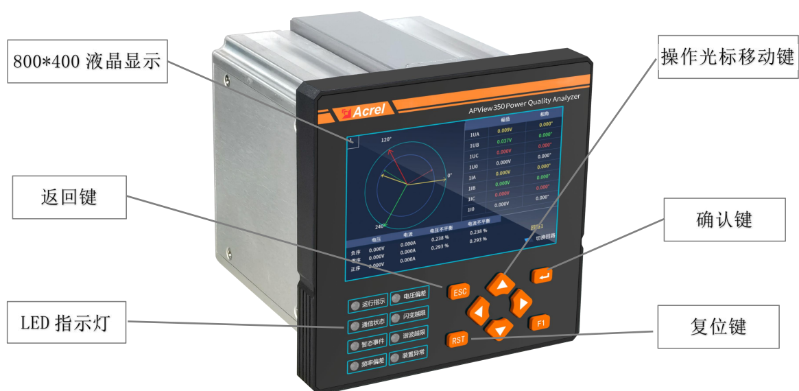
图 4.1 前面板说明
