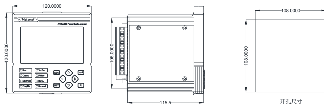
图 3.1 外形及开孔尺寸图
