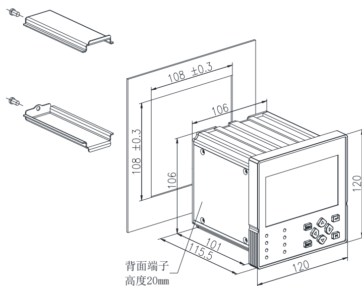
图 3.2 安装示意图
