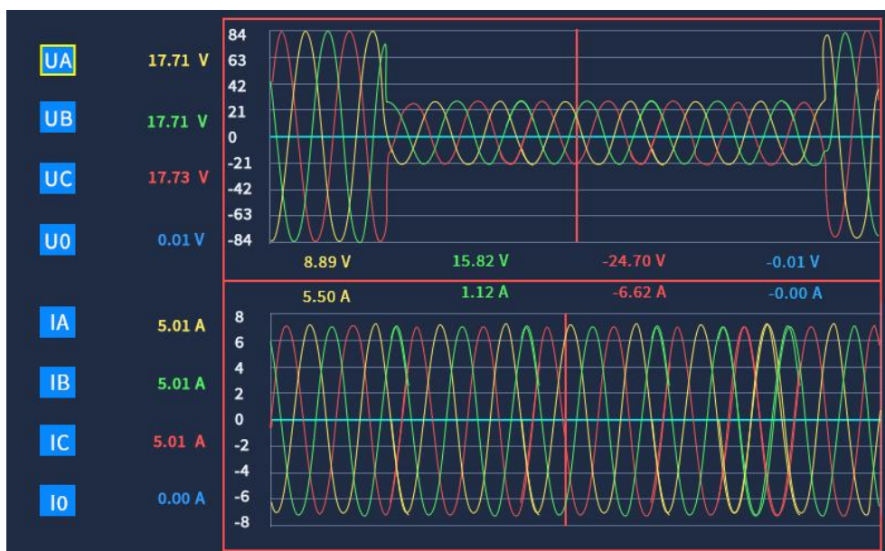
图 4.24(b) 电压暂降波形
