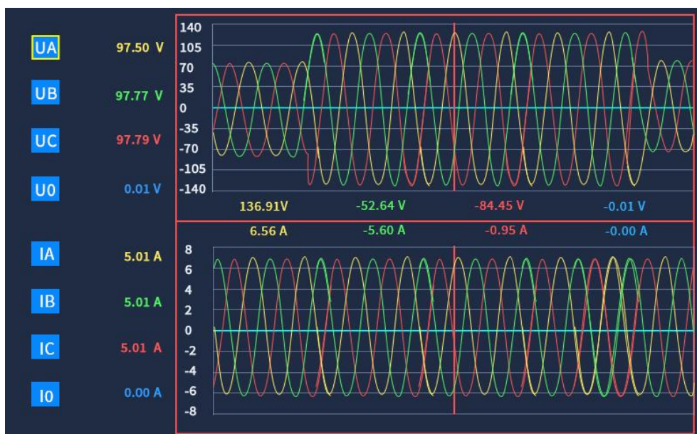
图 4.25(b) 电压暂升波形
