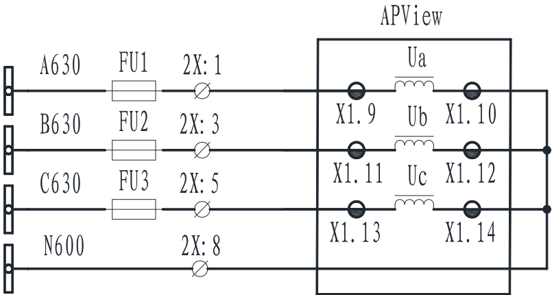
图 3.7 3PT 电压接线 Fig. 3.7 3PT Voltage wiring
