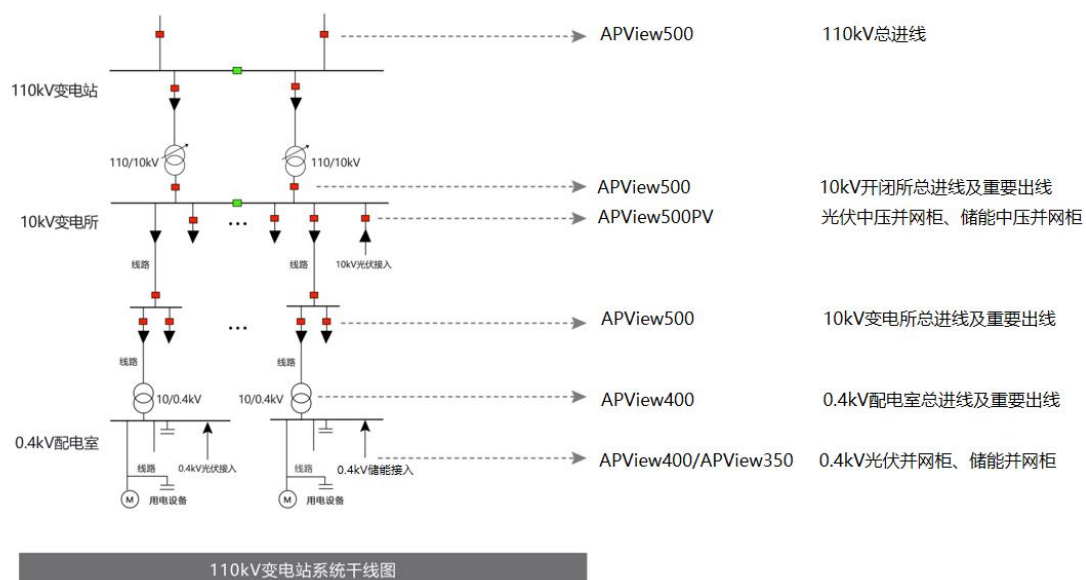
图 4.26 110kV 供电系统 APView 配置图 Fig. 4.26 APView configuration
