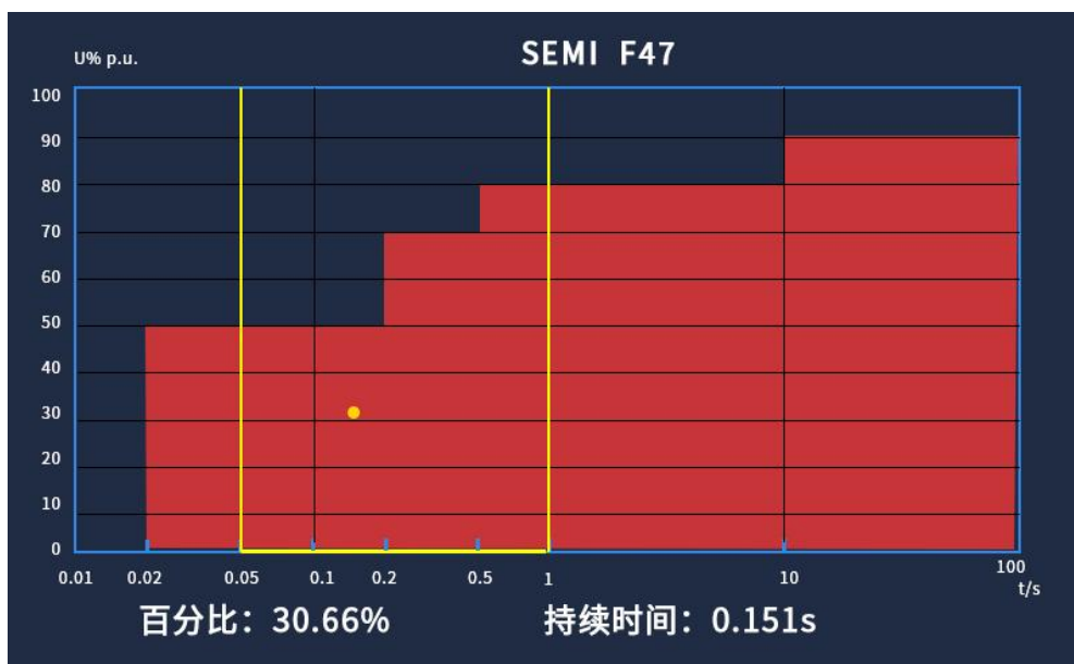
图 4.28(b) SEMI F47 容忍度曲线
