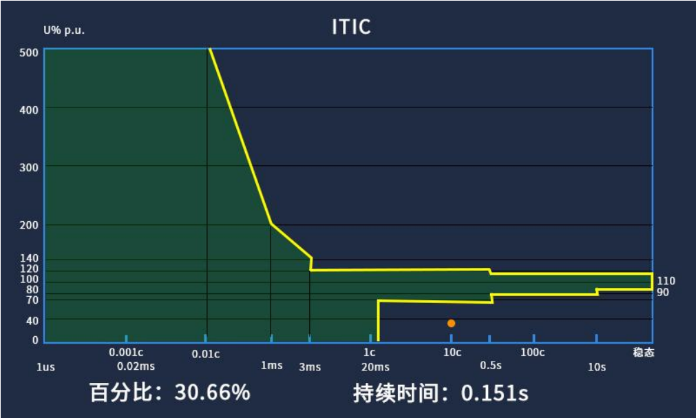
图 4.28(a) ITIC 容忍度曲线
