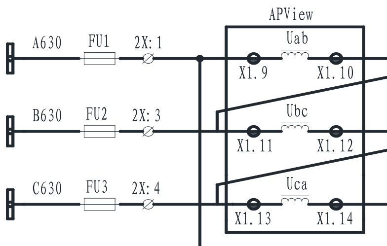
图 3.8 2PT 电压接线 Fig. 3.8 2PT Voltage wiring
