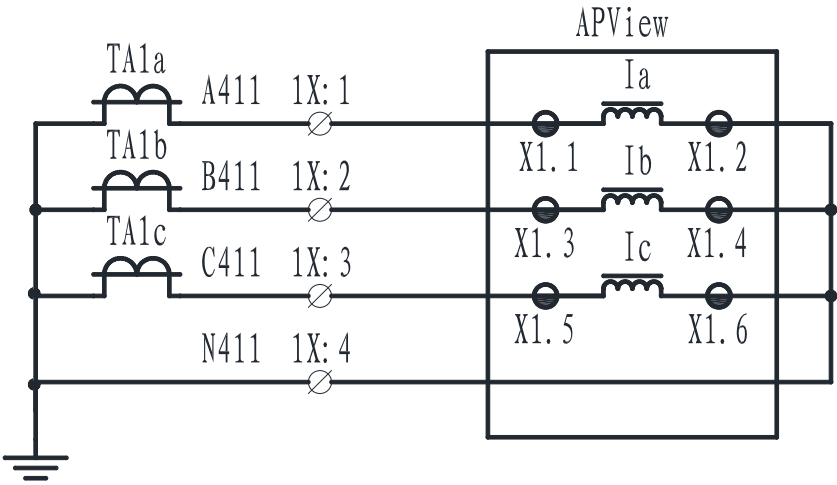
图 3.5 3CT 电流接线 Fig. 3.5 3CT Current wiring
