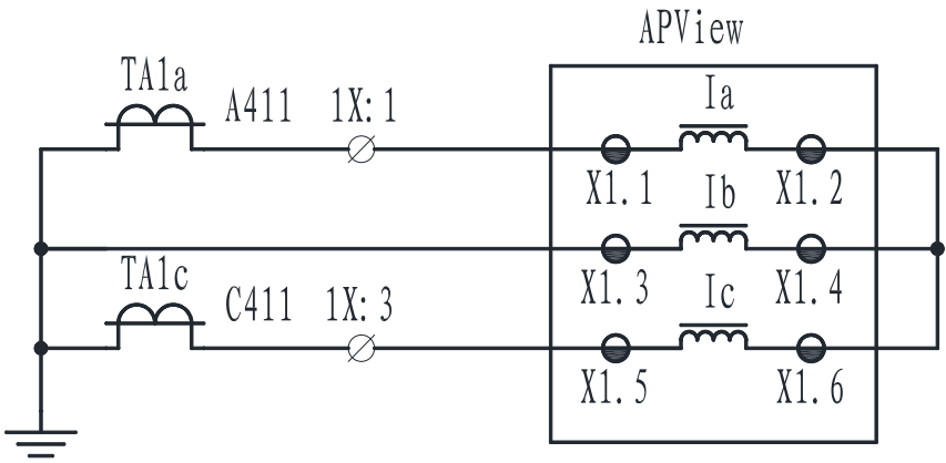
图 3.6 2CT 电流接线 Fig. 3.6 2CT Current wiring
