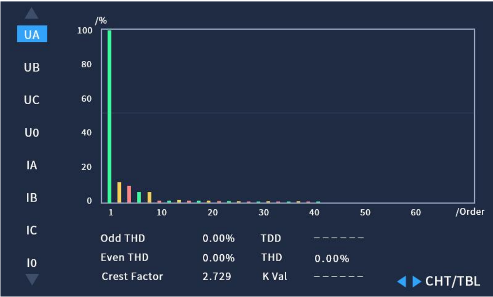
图 4.15 谐波柱状图
