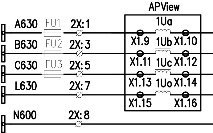
图 3.7 3PT 电压接线 Fig. 3.7 3PT Voltage wiring
