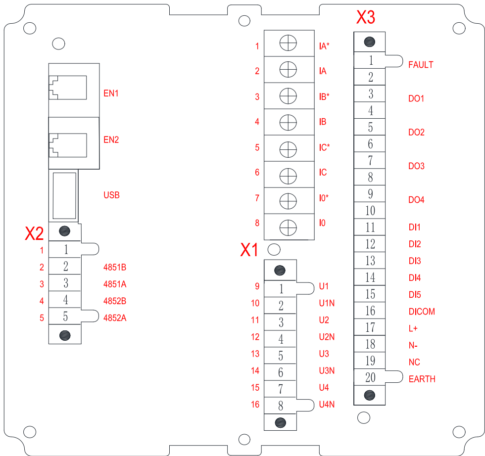
图 3.3 背部端子图
