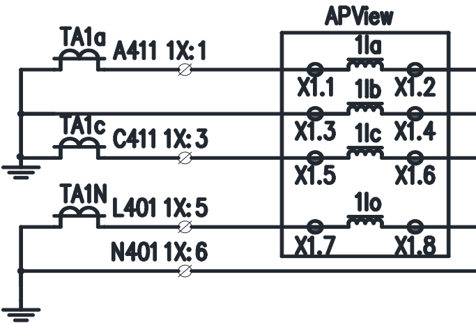
图 3.6 2CT 电流接线 Fig. 3.6 2CT Current wiring
