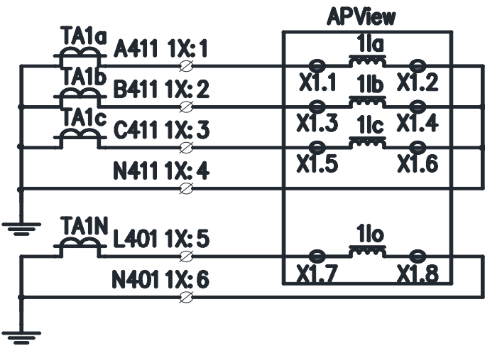
图 3.5 3CT 电流接线 Fig. 3.5 3CT Current wiring
