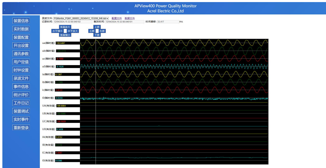
图 1.5 波形界面
