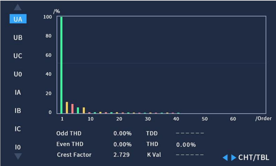
图 4.13 谐波柱状图
