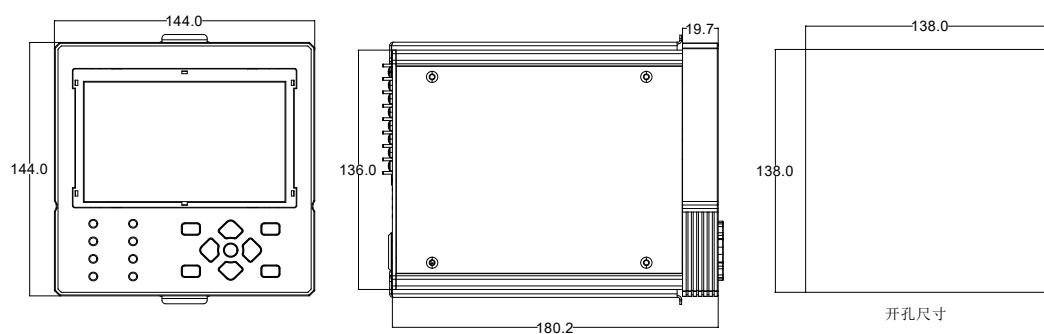
图 3.1 外形及开孔尺寸图
