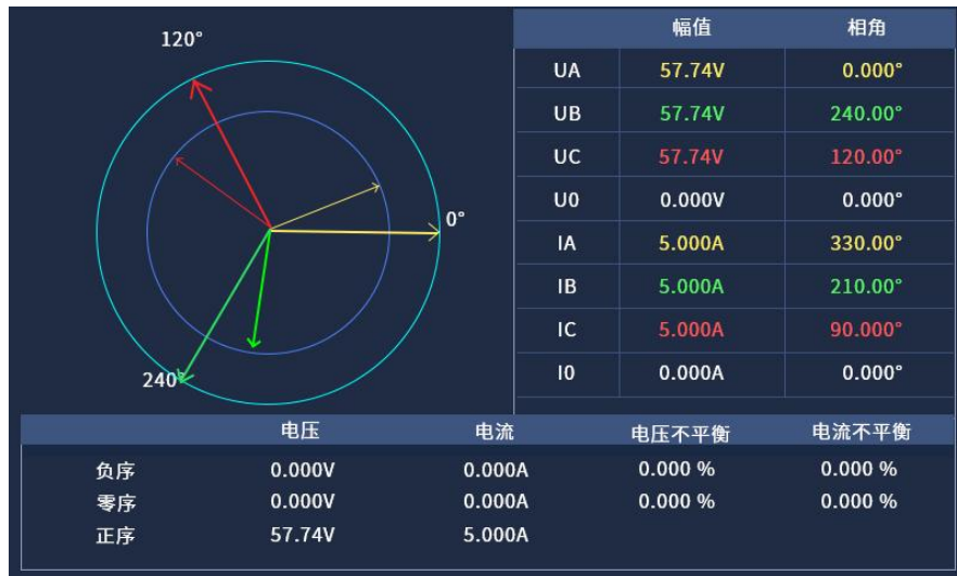
图4.8 矢量图
