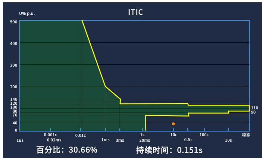
图 4.26(a) ITIC 容忍度曲线
